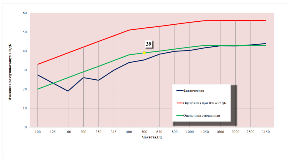
Рис. 3 Спектр изоляции фрагмента перегородки «базовая конструкция + бескаркасная конструкция для дополнительной звукоизоляции стен (вариант №4)»
