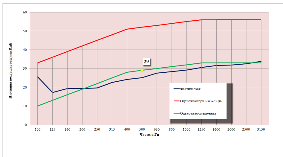
Рис. 1 Спектр базовой плиты (МДФ)
